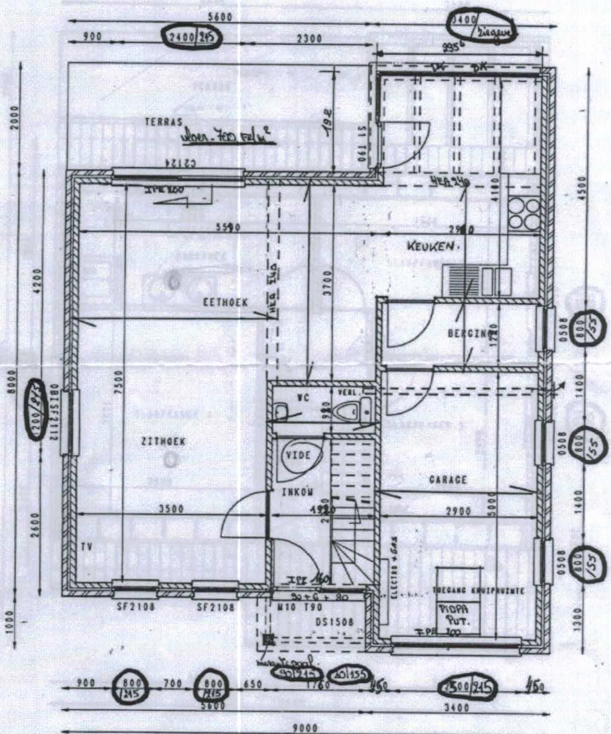
GRONDPLAN
