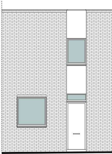
Voorgevel 1/100
