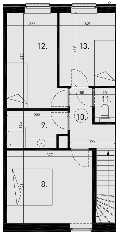
Verdieping 1/100
