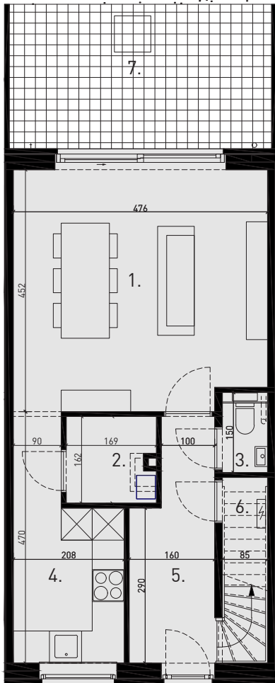
Gelijkvloers 1/100
