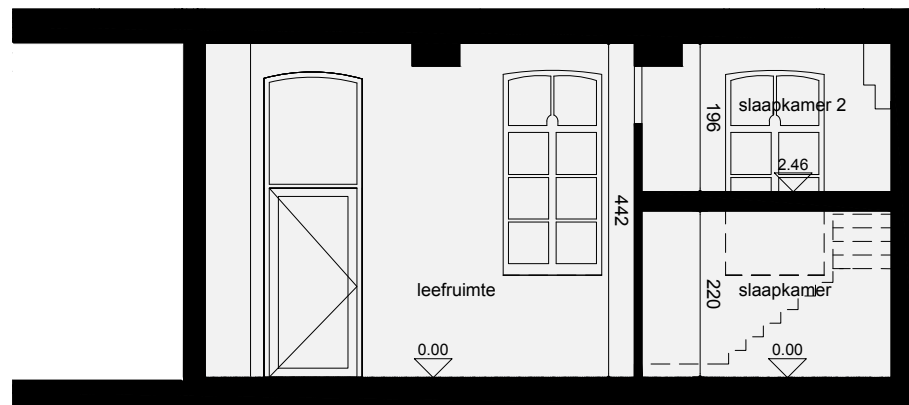
SNEDE SCHAAL 1:100
