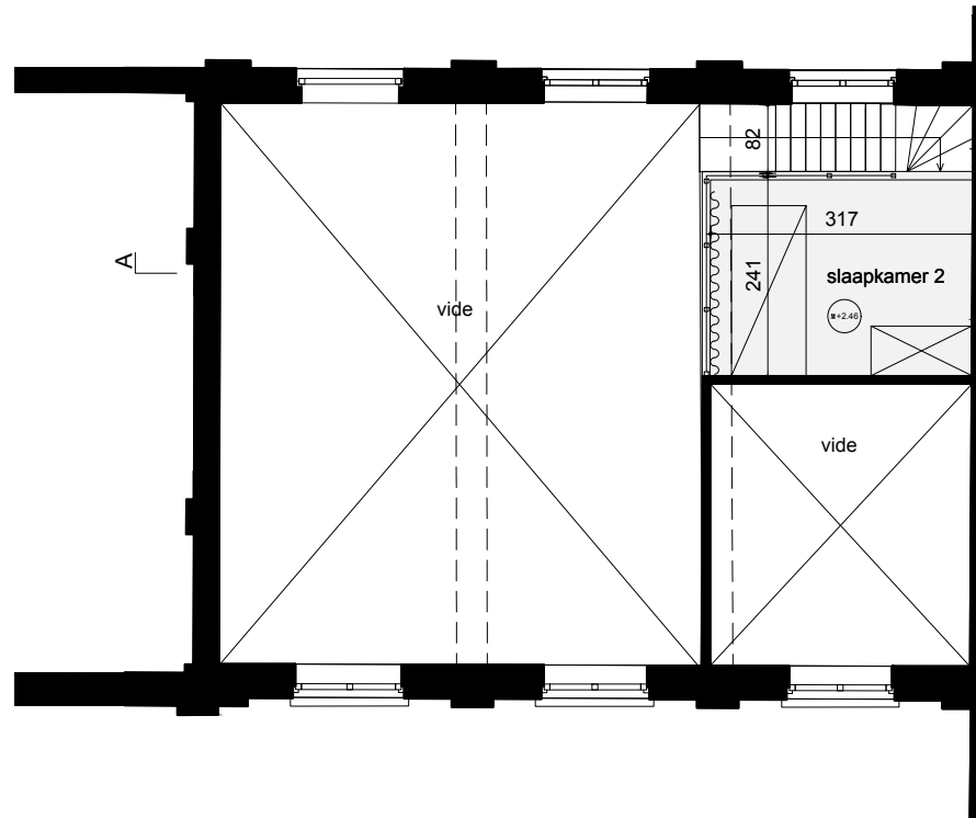
NIVEAU +0 MEZZANINE SCHAAL 1:100
