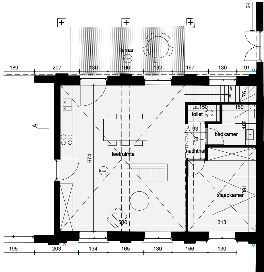
NIVEAU +0 SCHAAL 1:100
