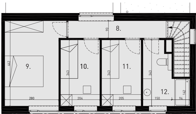
Verdieping 1/100
