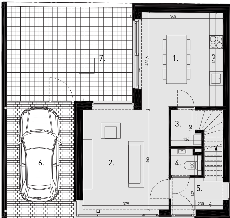
Gelijkvloers 1/100
