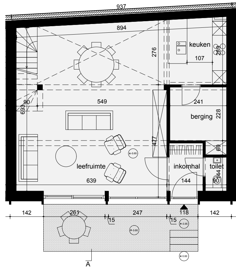
NIVEAU +0 SCHAAL 1:100
