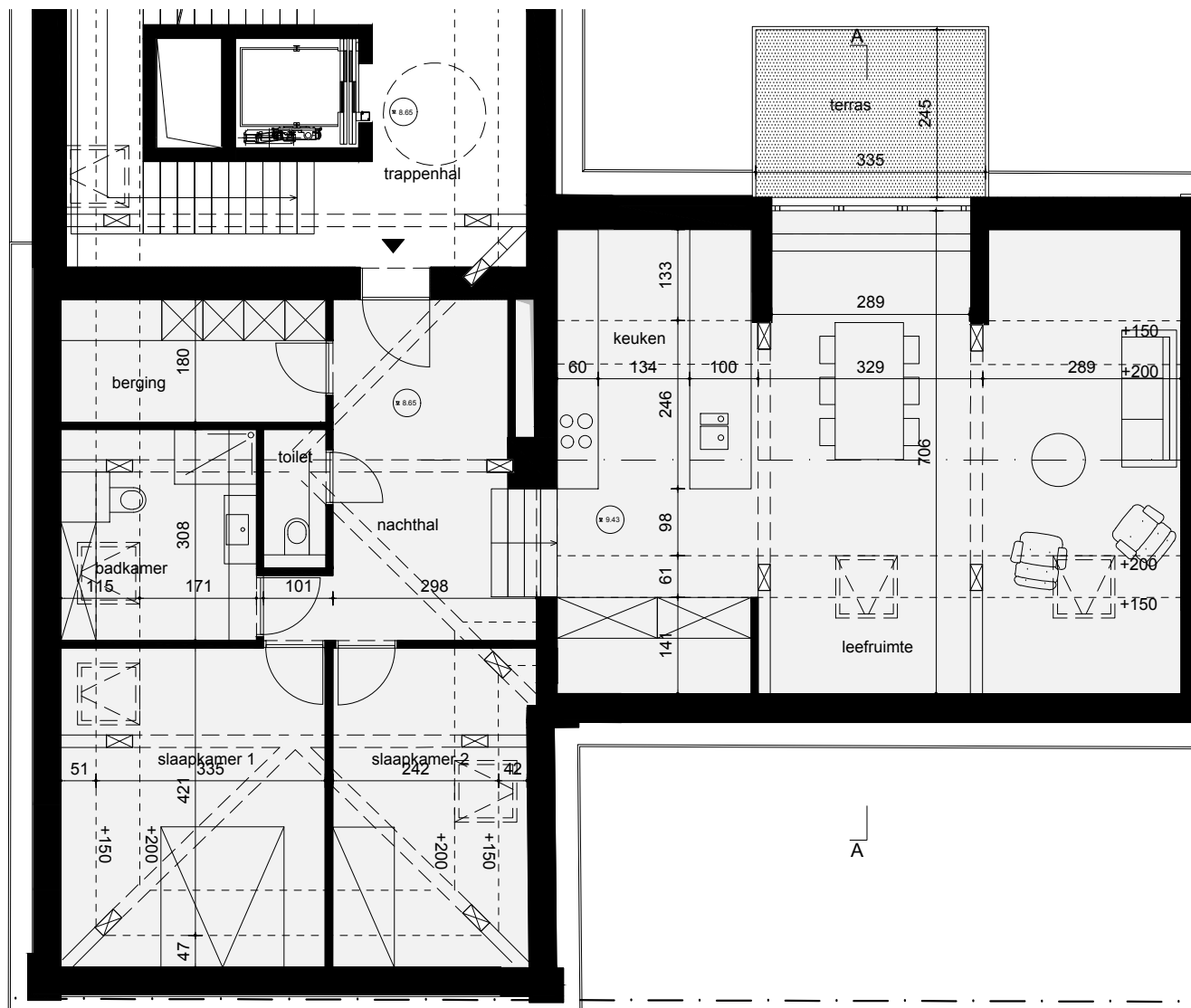
NIVEAU +2 SCHAAL 1:100
