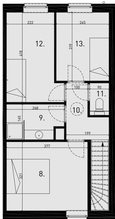
Verdieping 1/100
