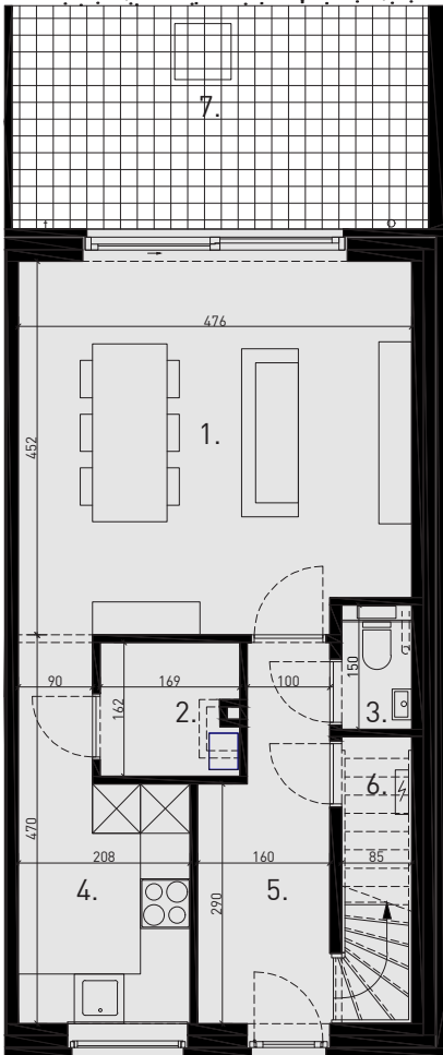
Gelijkvloers 1/100
